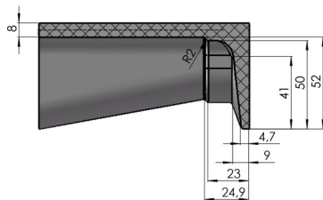
SECTION B SCALE 1 : 1.5
