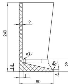
SECTION D SCALE 1 : 2
