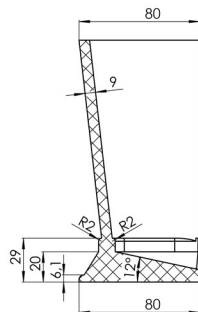
SECTION C SCALE 1 : 2
