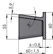
SECTION F SCALE 1 : 2
